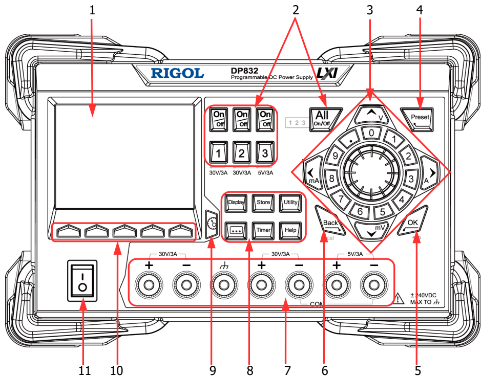
图 1-3 DP832 前面板
